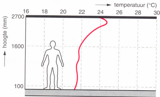
5 gestuwde lucht tegenover de gevel 5 vol/h en 1,5 m/s
