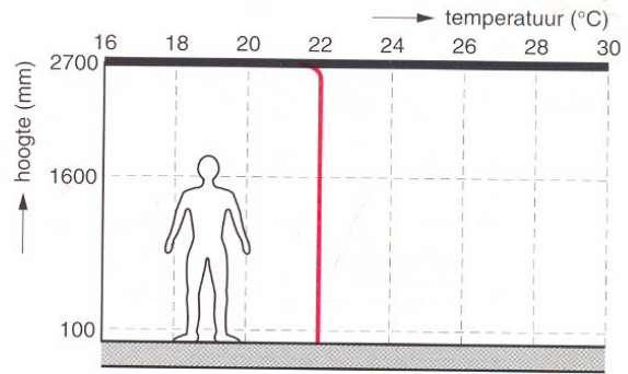
2 warm water met enkel paneel onder het raam
